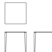
6002 - 6102 L.90cm P.90cm H.76cm W.35 1/2" D.35 1/2" H.30"
